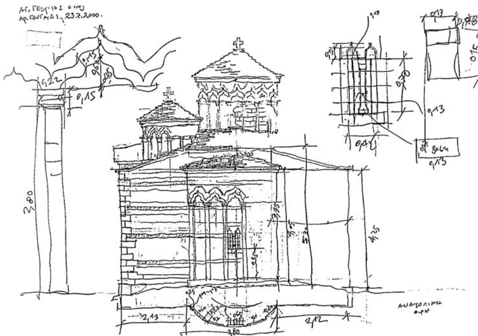
Αποτύπωση Ανατολικής Όψης
