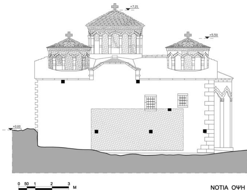
Νότια όψη, Αποτύπωση
