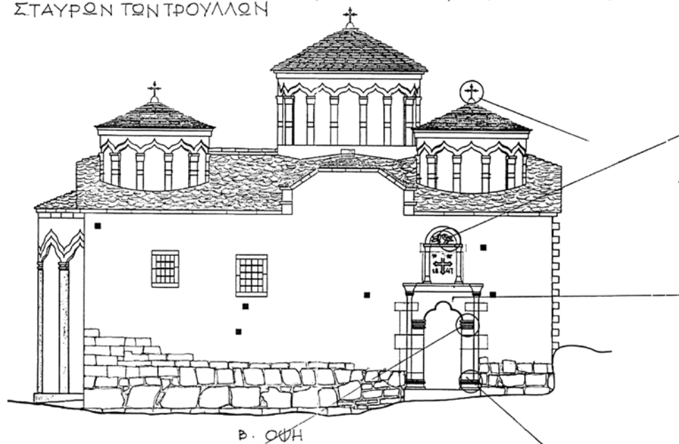
Αποτύπωση Βόρειας Όψης
