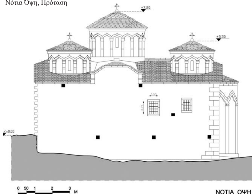
Νότια Όψη, Πρόταση
