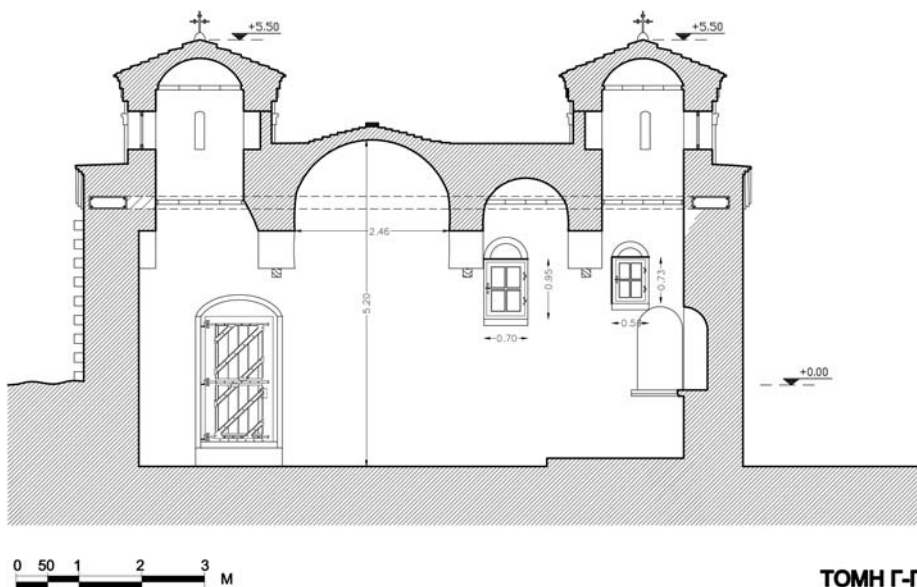
Τομή Γ-Γ, Πρόταση
