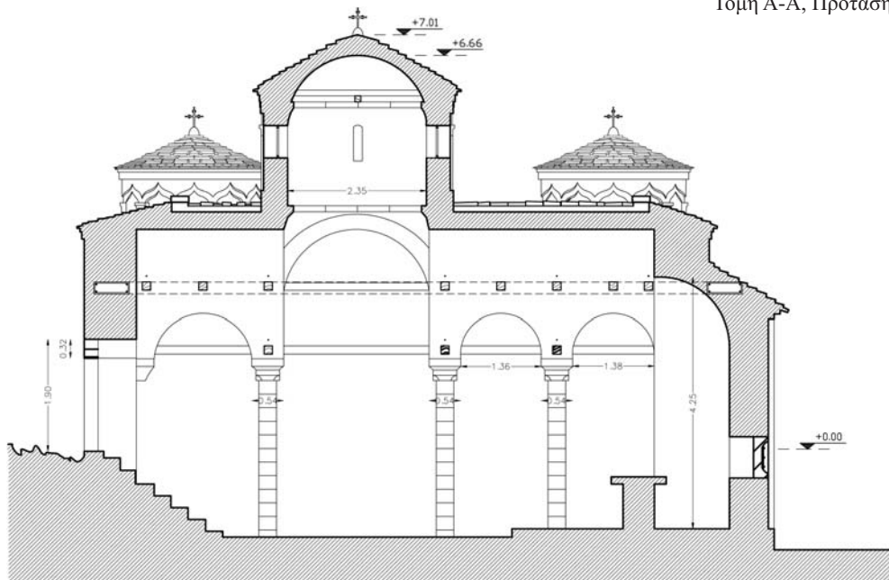
Τομή Α-Α, Πρόταση
