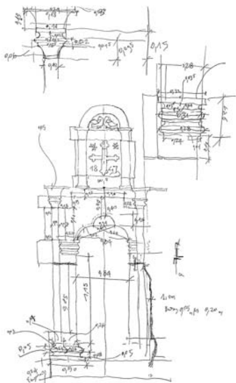
Αποτύπωση Κυρίας εισόδου
